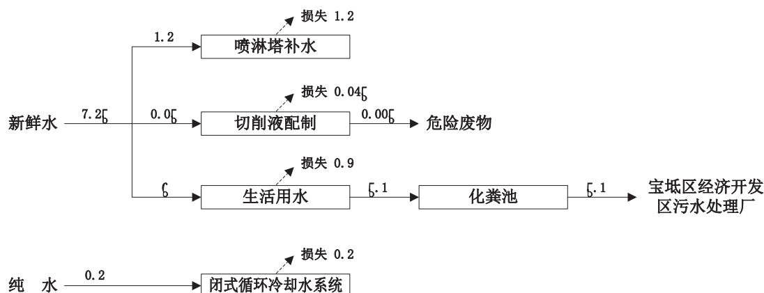
图 2.7-1 水平衡图 (单位: \text{m}^3/\text{d} )
