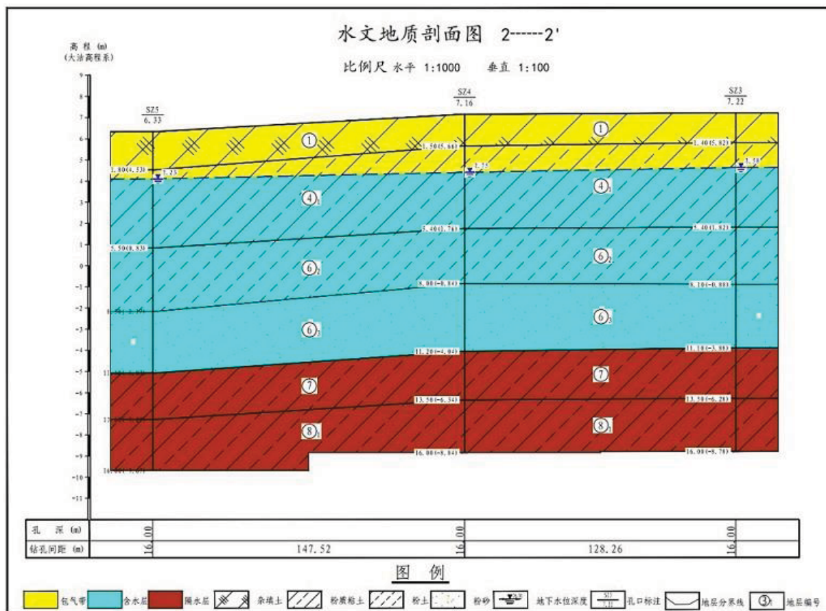
图 3.2-2 2—2' 水文地质剖面图
