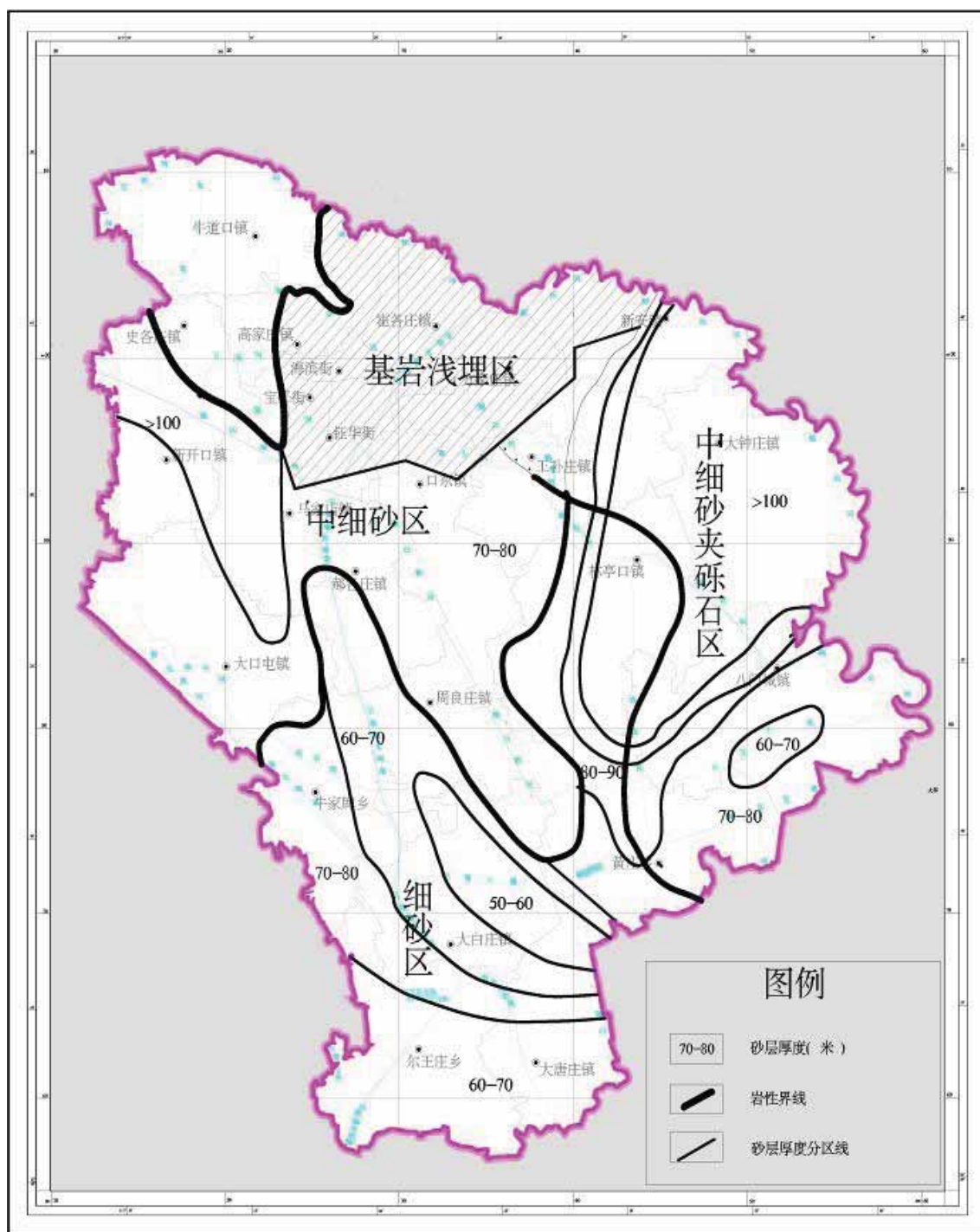
图 3.1-2 宝坻区深层砂层分布图（250-260m 埋深内）
