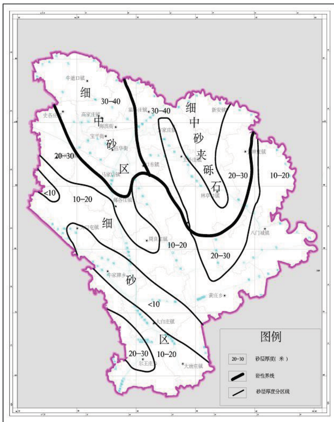
图 3.1-1 宝坻区浅层砂层分布图（70-80m 埋深内）
