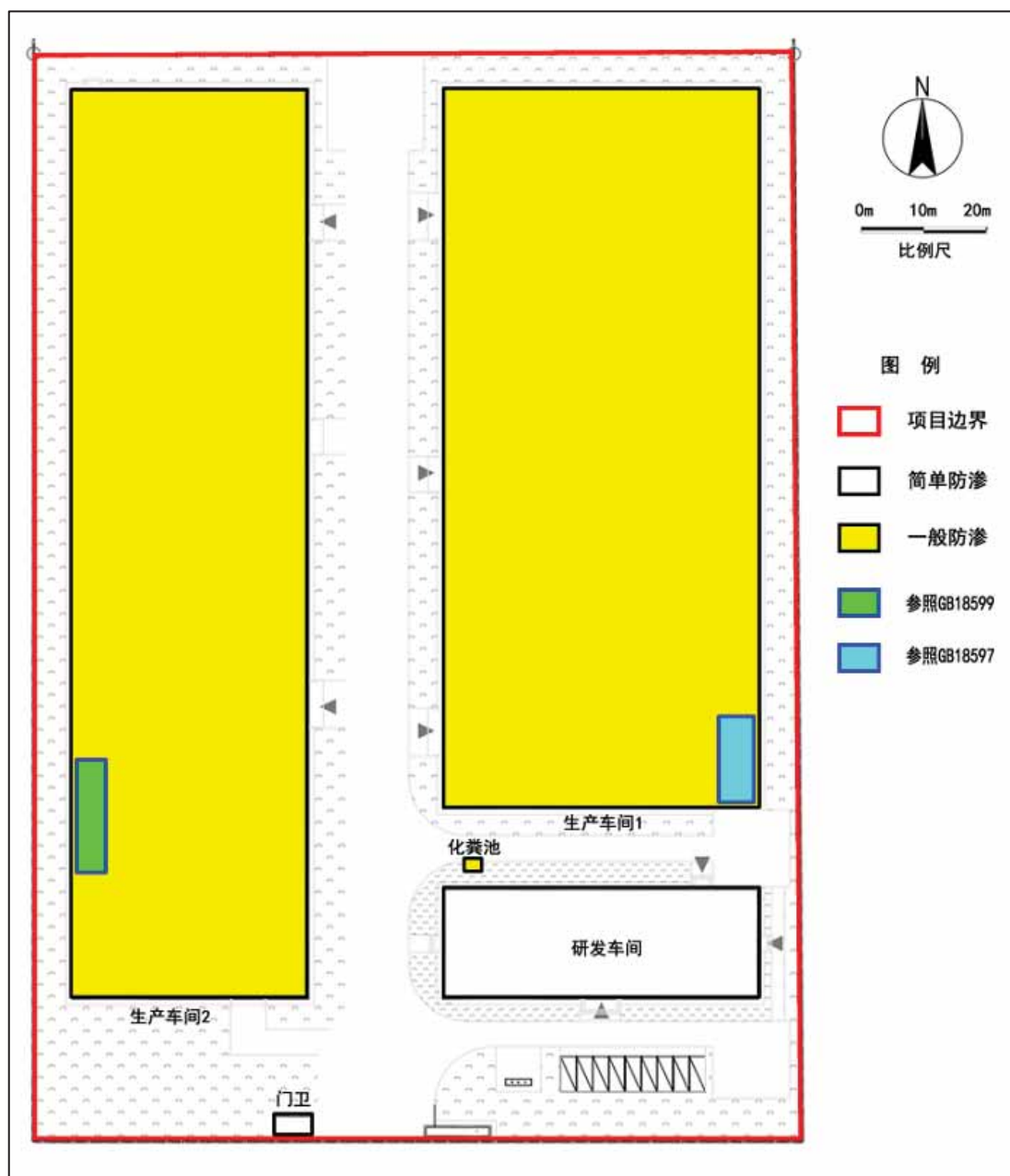
图 12.6-1 防渗分区图
