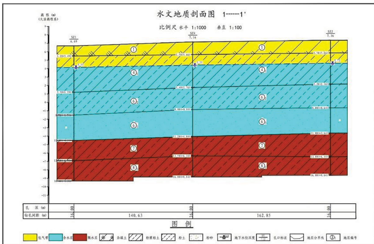
图 3.2-1 1—1' 水文地质剖面图
