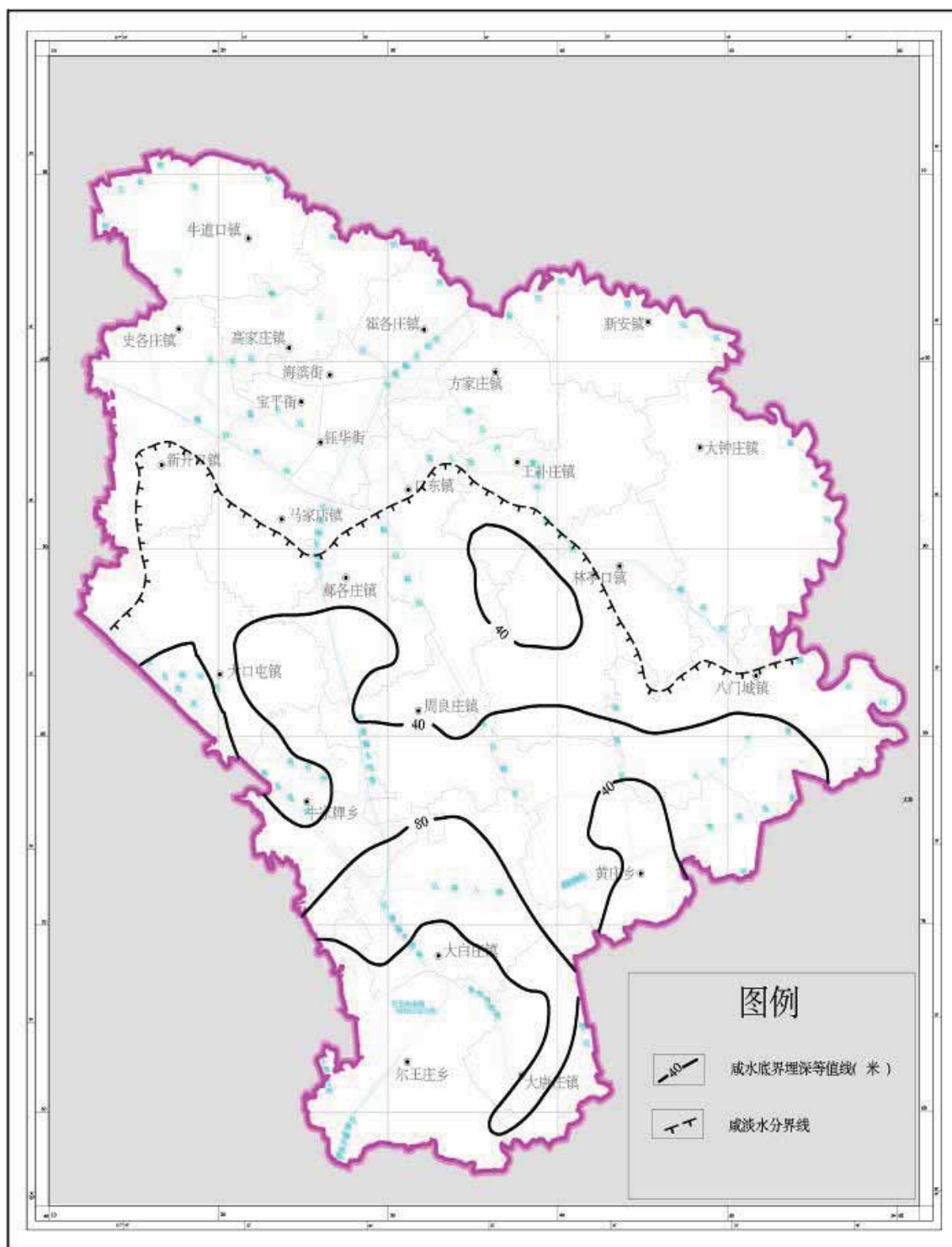
图 3.1-3 宝坻区咸水底界埋深图
